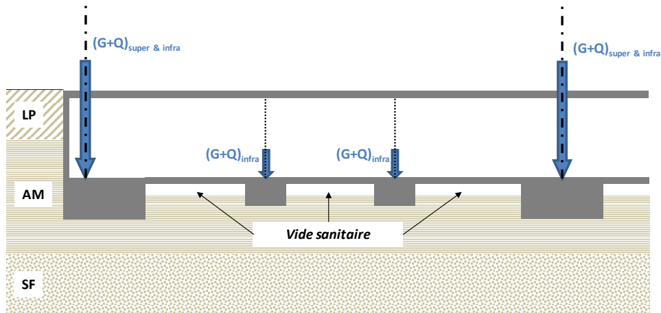
Figure 6. Conception des fondations du bâtiment 1
