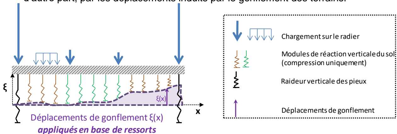
Figure 9. Sous-modèle structurel du radier
