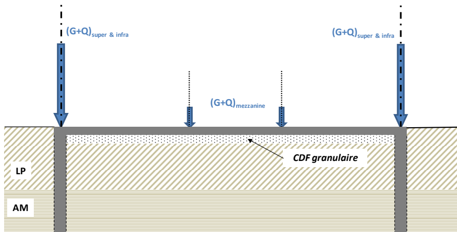
Figure 7. Conception des fondations des bâtiments 2 à 8
