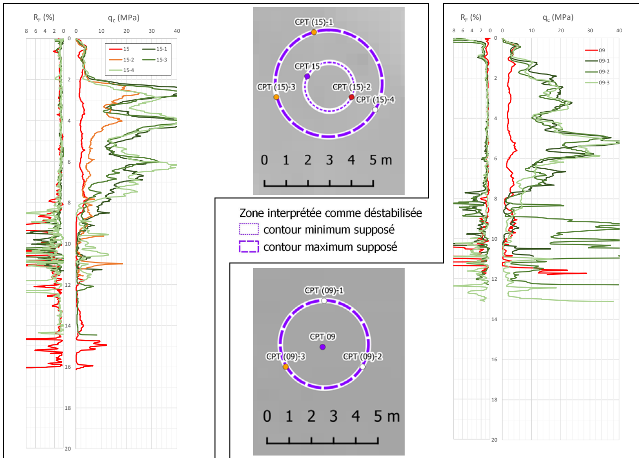
Figure 5 : Fontis karstiques, anciens ou en cours, repérés au niveau du CPT 15 et du CPT 9
