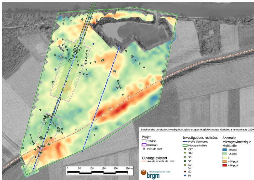
Figure 3 : Investigations réalisées de 2006 à 2019 avec, en fond, les résultats microgravimétriques
