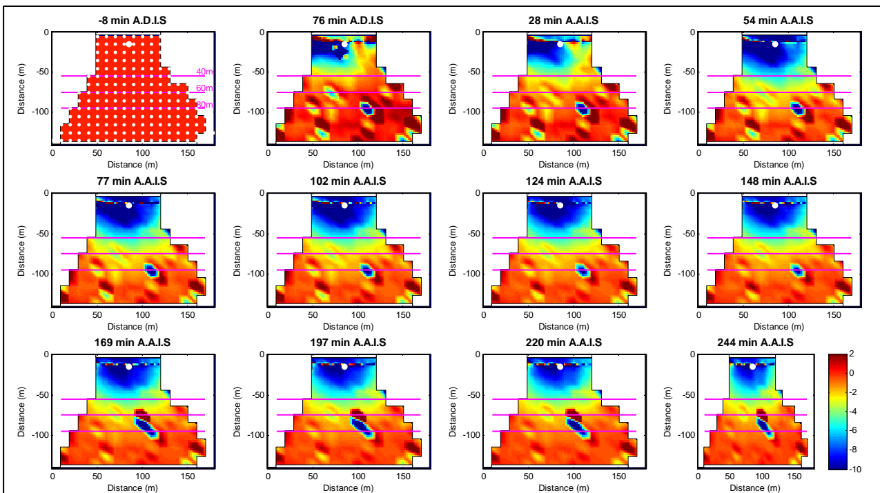
Figure 6 : Cartes de conductivité de suivi du traçage salin
