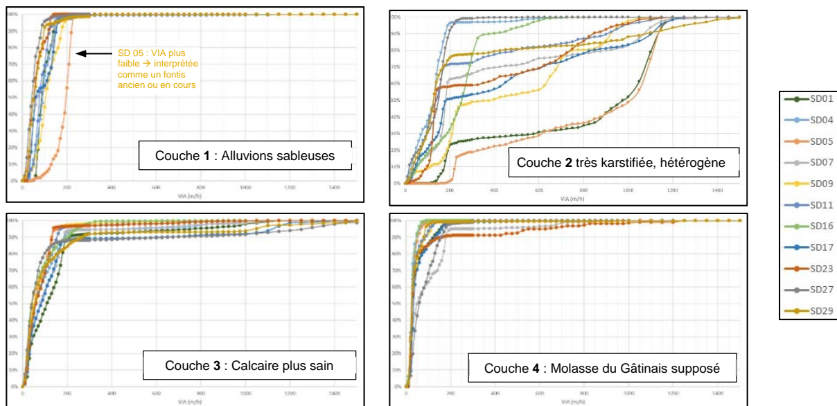
Figure 4 : Traitement statistique du paramètre VIA enregistré par les sondages destructifs
